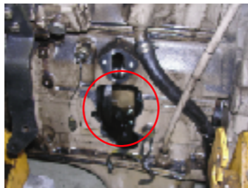
假的活塞导致发动机拉缸，第三缸缸体被打破
